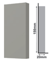
Sócalo 183 Cinza Glacial Glacial Gray Plinth Block Zócalin Gris Glacial 70 x 150 x 20mm Cód. | Code - 22392
