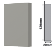
Sócalo 178 Cinza Glacial Glacial Gray Plinth Block Zócalin Gris Glacial 80 x 120 x 20mm Cód. | Code - 22396
