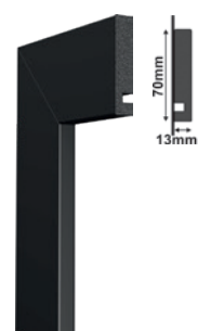
3451 GN/Black Black Architrave Contramarco Negro Cód. | Code - 21366
