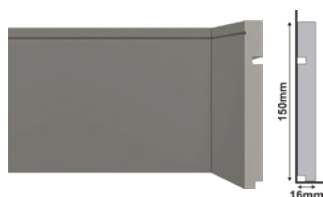
518 RP Cinza Titanium Titanium Gray Skirting Board Zócalo Gis Titanio
