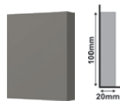
Sócalo 177 Cinza Titanium Titanium Gray Plinth Block Zócalin Gris Titano 80 x 100 x 20mm Cód. | Code - 22395
