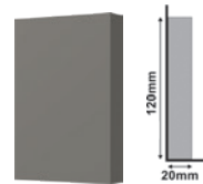
Sócalo 178 Cinza Titanium Titanium Gray Plinth Block Zócalin Gris Titano 80 x 120 x 20mm Cód. | Code - 22397
